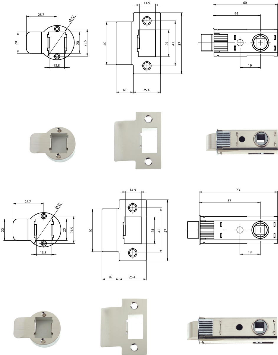
Tubular Latch
